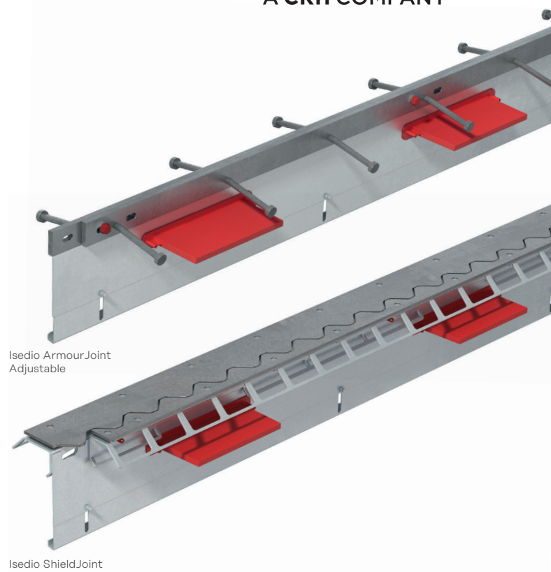
Ise dio ArmourJoint Adjustable
