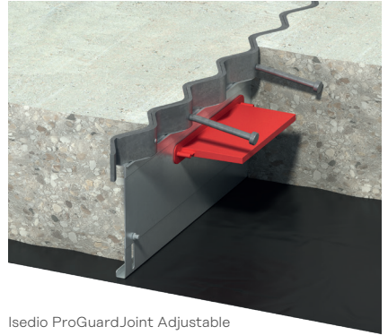
Isedio ProGuardJoint Adjustable
